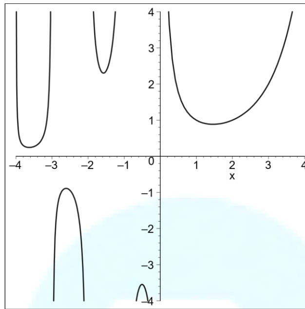
\Gamma(x) function
