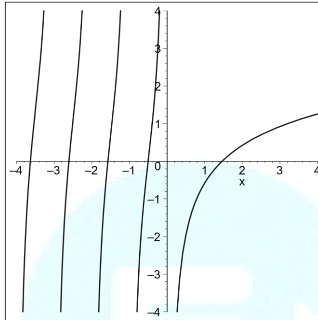
(digamma)
